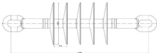
CRTEŽ 4 – ŠTAPNI IZOLATOR SA KUĆIŠTEM OD SILIKONIZOVANE GUME SA POJAČANOM ELEKTRIČNOM IZOLACIJOM 24 kV
